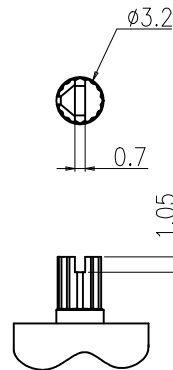
ACTUATOR
