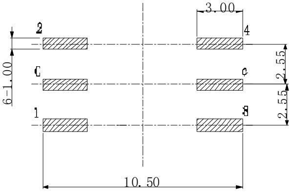
PCB布局图 PCB LAYOUT
